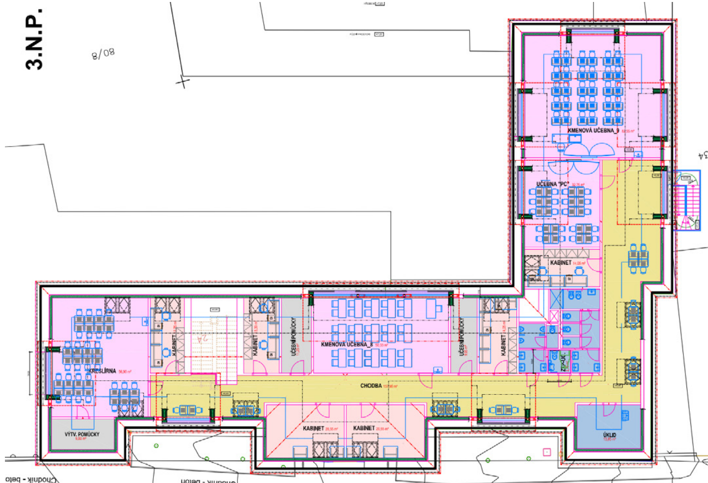
Představa projektanta o uspořádání budoucího druhého patra hlavní budovy základní školy
